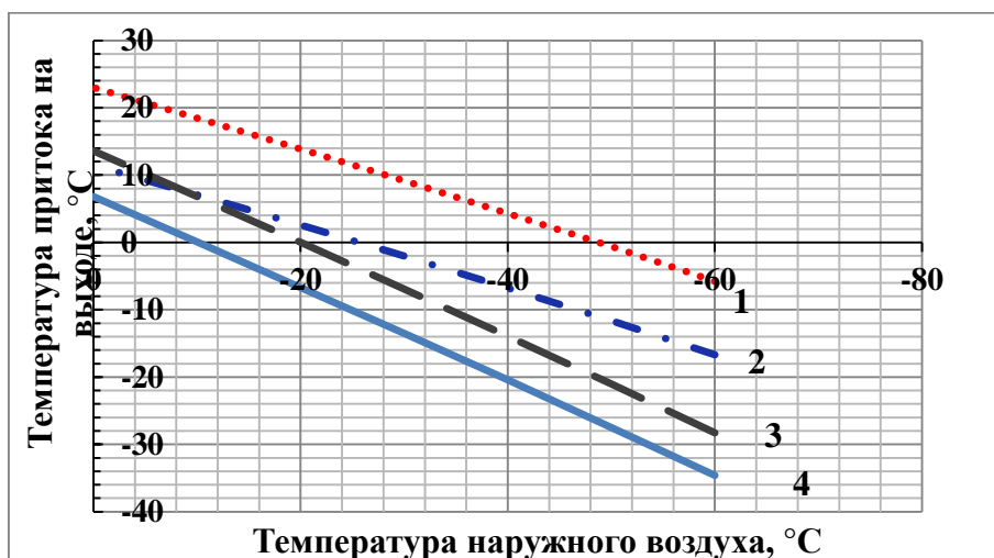
Рис. 1. Изменение температуры притока на выходе при: 1 – G_v/G_n=2 и t_1' = 40^{\circ}\text{C} ; 2 – G_v/G_n=2 и t_1' = 20^{\circ}\text{C} ; 3 – G_v/G_n=1 и t_1' = 40^{\circ}\text{C} ; 4 – G_v/G_n=1 и t_1' = 20^{\circ}\text{C}
