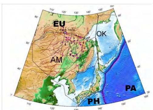
Рис.1. Группирование эпицентров землетрясений вдоль северо-восточного сегмента Амурской коровой плиты.
