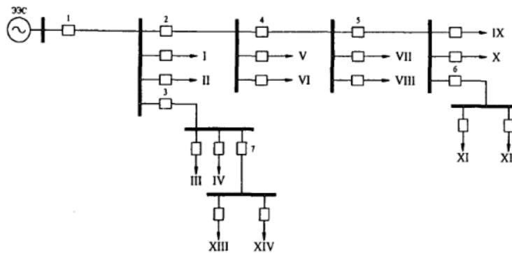
Рисунок 1 — Схема сети
