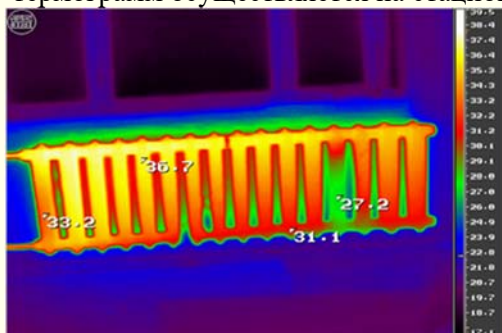
Рис. 1. Термограмма отопительного радиатора
