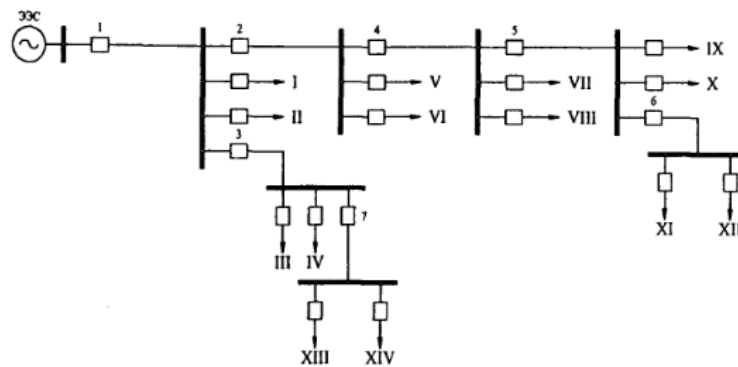
Рисунок 1 — Схема сети
