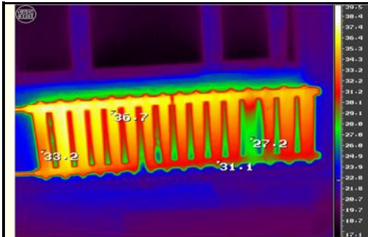
Рис. 1. Термограмма отопительного радиатора
