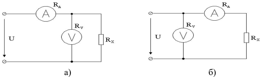
Рис. 1. Схемы измерения сопротивления методом амперметра и вольтметра:
